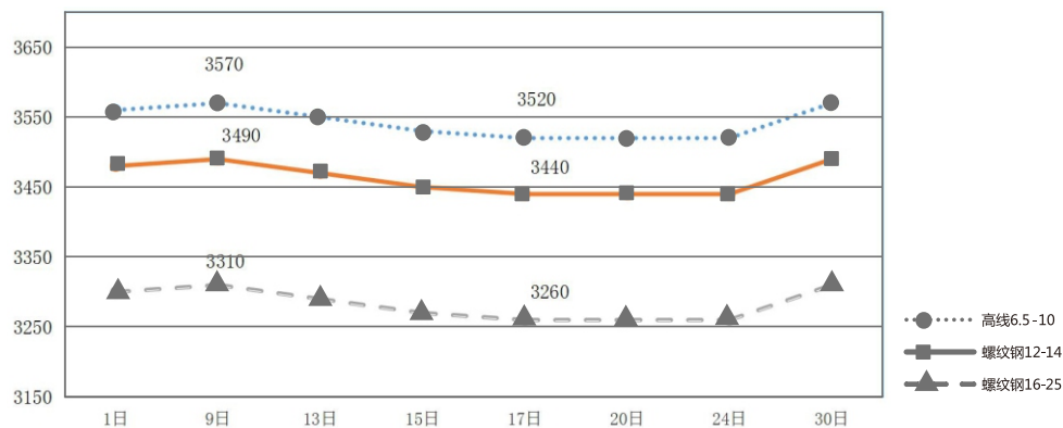
2025年10月中心城区主要钢材趋势图
