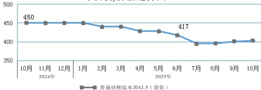
2024年10月—2025年10月中心城区普通硅酸盐水泥42.5 (袋装)价格趋势图
