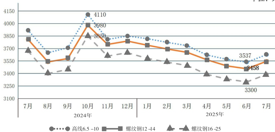
2024年7月—2025年7月中心城区主要钢材价格趋势图
