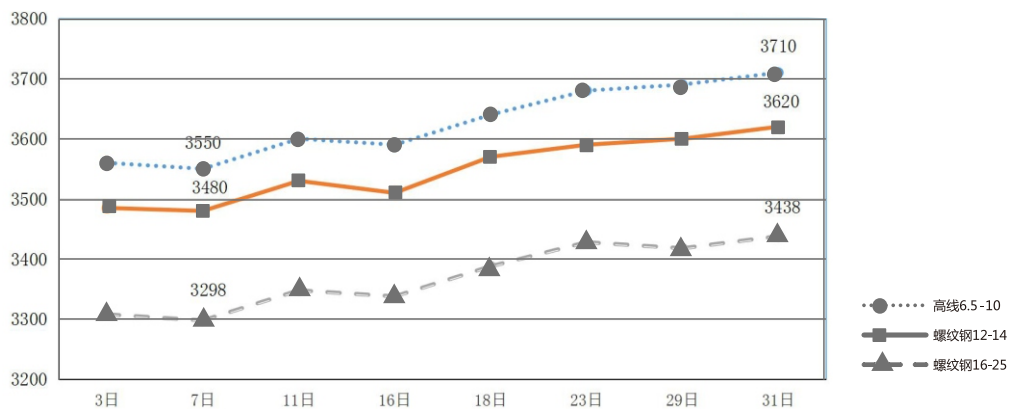
2025年7月中心城区主要钢材趋势图
