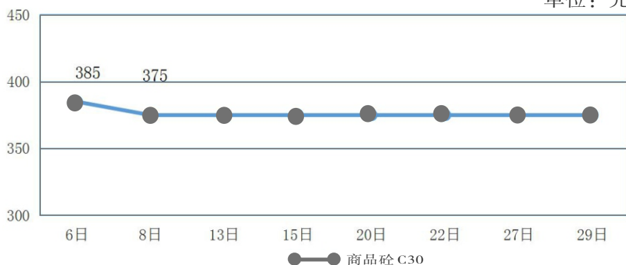
2025年7月中心城区商品砼C30 价格趋势图
