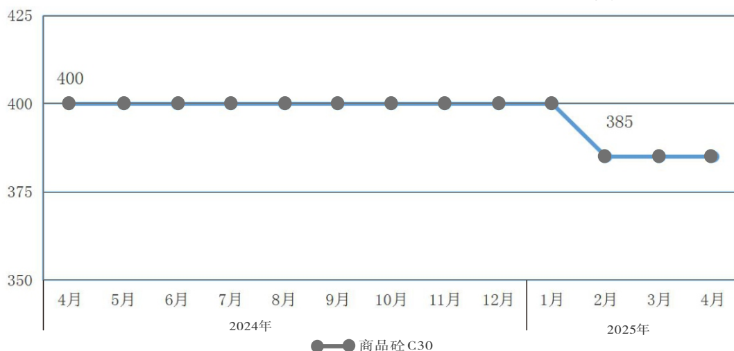
2024年4月—2025年4月中心城区商品砼 C30 价格趋势图
