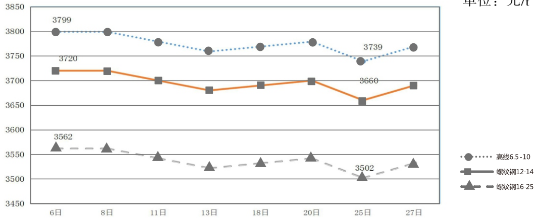
2025年2月中心城区主要钢材趋势图
